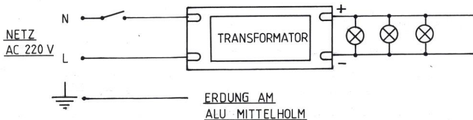
⑦ SCHALTPLAN BELEUCHTUNG PICCO SPOT
