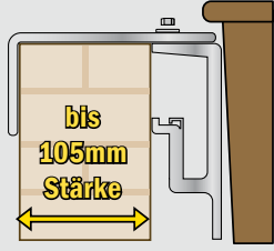
Betonbalkon
