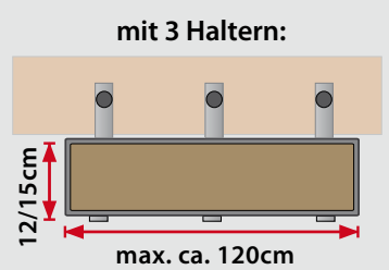
Edelstahlgeländer
