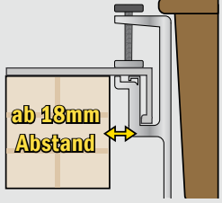
Fensterbankprofile
